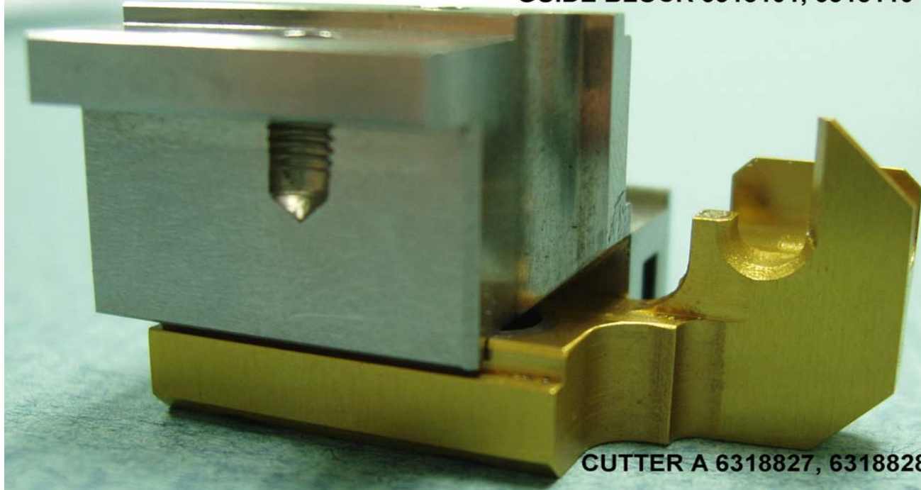
GUIDE BLOCK 6318101, 6318110
